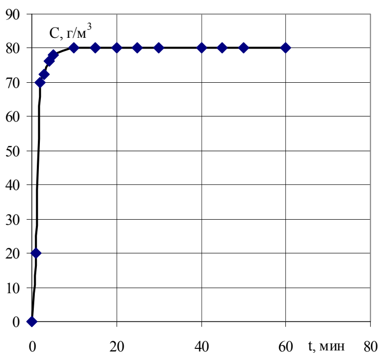
Рис. 5 Зависимость концентрации озона от времени работы озонатора.
