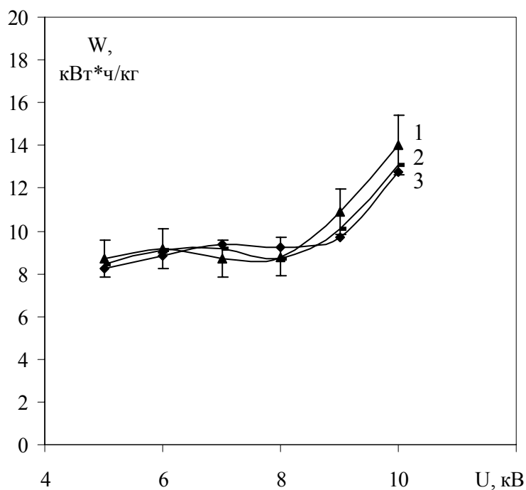
Рис 4. Зависимость удельных энергозатрат от напряжения на разрядной ячейке для следующих значений расхода кислорода 0.043 (1), 0.058 (2), 0.072(3) м 3 /ч.
