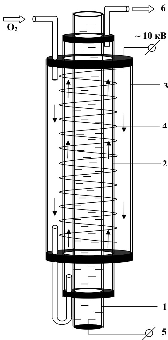
Рис.1 Озолирующая ячейка. 1 – Центральная труба. 2 – Промежуточная труба. 3 – Корпус установки. 4 – Высоковольтный электрод. 5 – Заземленный электрод. 6 – Патрубок для вывода озона.
