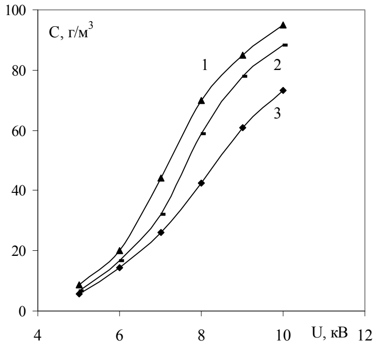
Рис 3. Зависимости концентрации озона от подводимого напряжения для различных значений расхода кислорода 0.043 (1), 0.058 (2), 0.072-(3) м 3 /ч.
